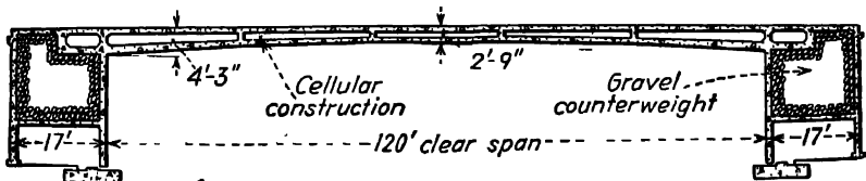
Fig. 354.—Longitudinal Section.
